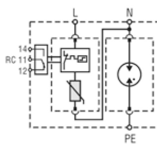
ETITEC T2 1+1 RC
