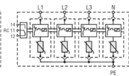
ETITEC T2 4+0 RC
