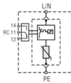
ETITEC T2 1+0 RC
